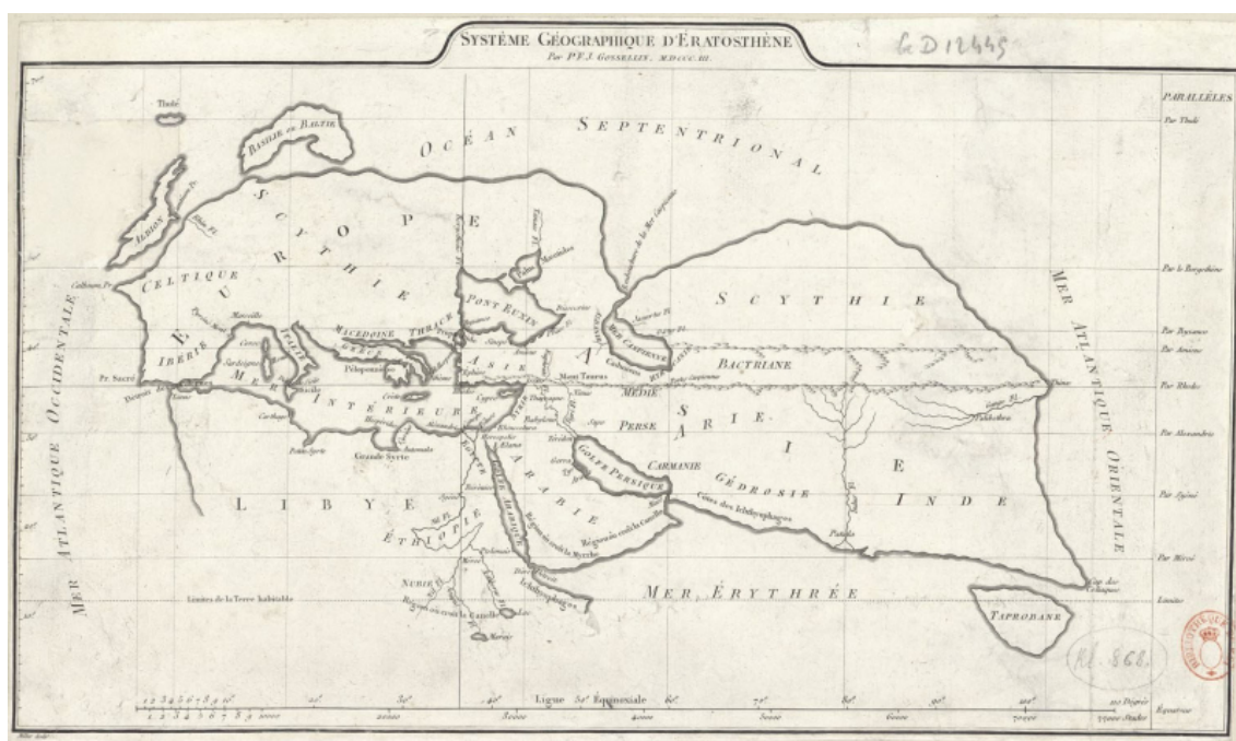
Figure 2. – Système géographique d'Eratosthène par Gosselin, 1803
